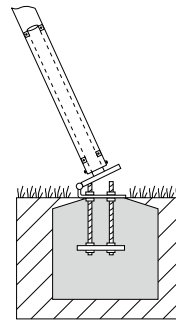
Kipphalterung aus Stahl mit Sicherheitsscharnier und Justierbolzen
